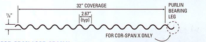
COR-SPAN / COR-SPAN X
